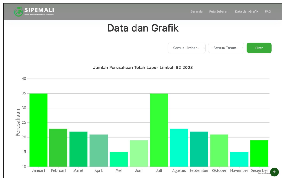
Gambar 4 Grafik Pelaporan
