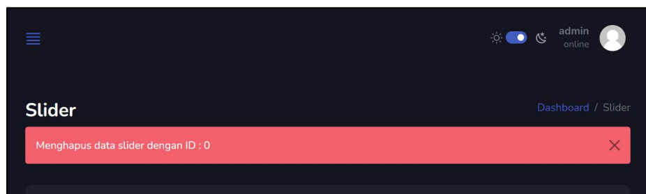
Gambar 58 Hapus Data
