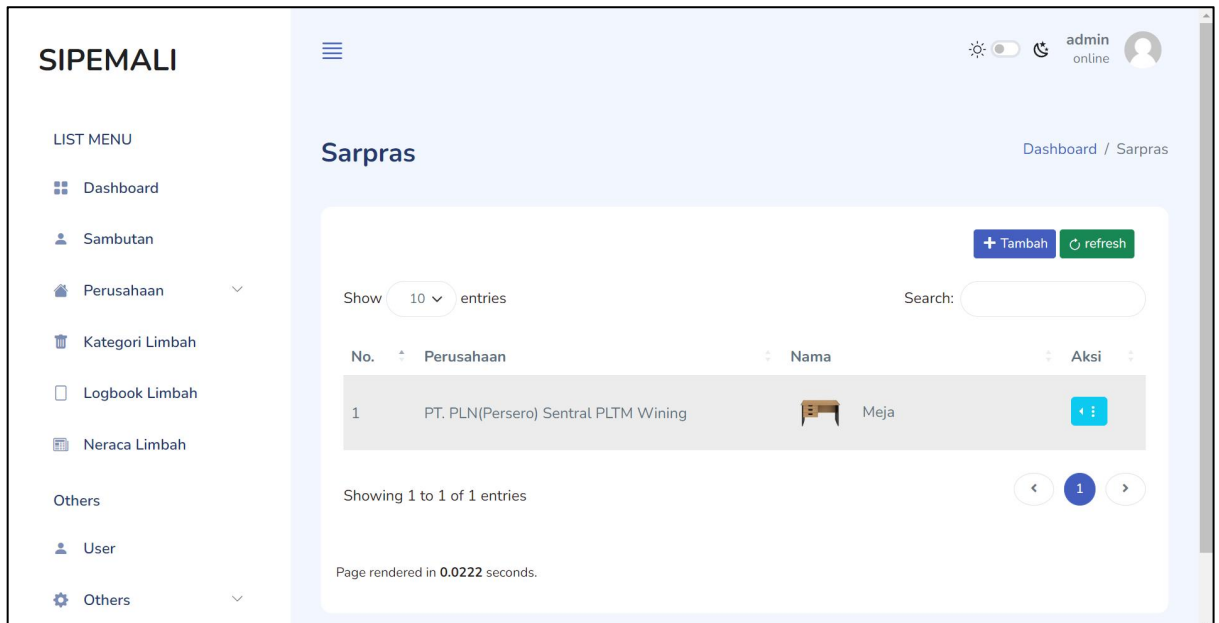
Gambar 26 Menu Sarpras
