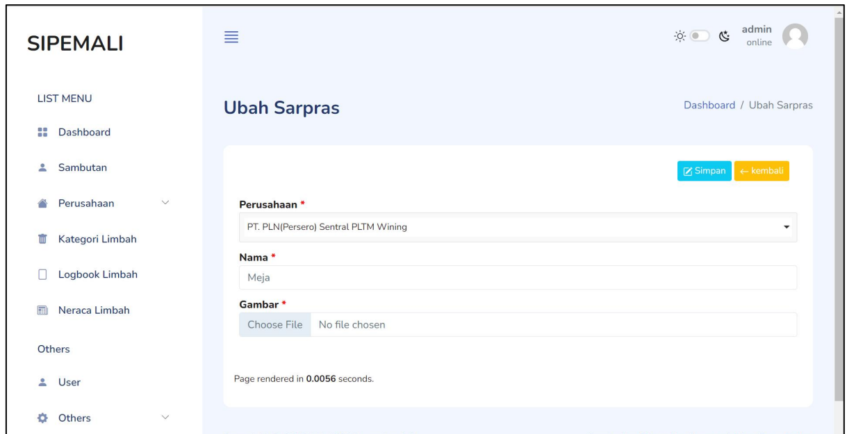
Gambar 30 Ubah Sarpras
