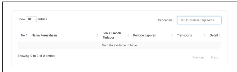
Gambar 5 Data Pelaporan
