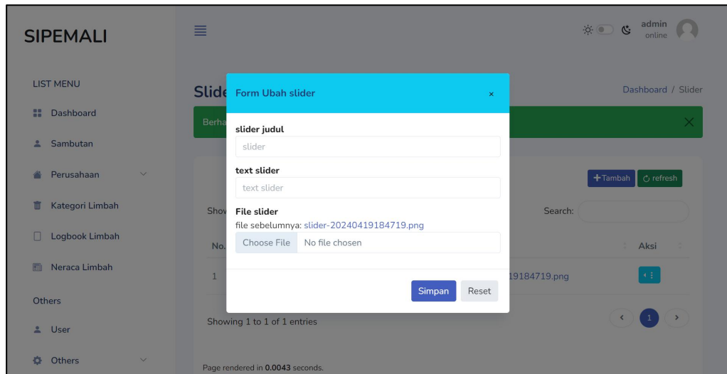
Gambar 57 Ubah Data
