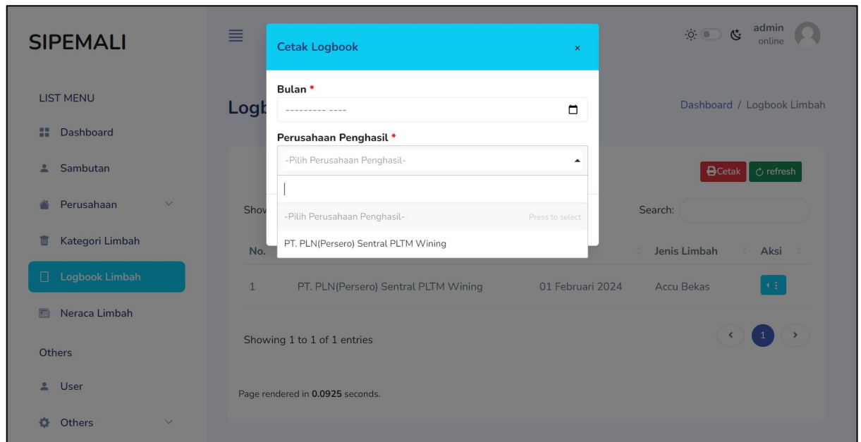
Gambar 39 Cetak Loogbook
