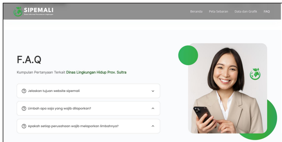
Gambar 10 Menu FAQ
