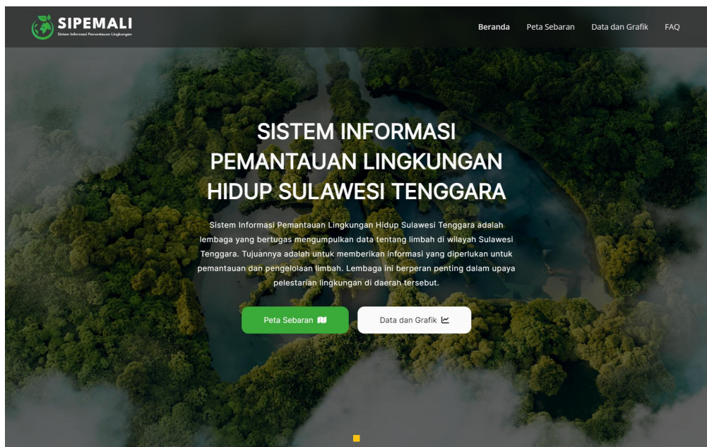
Gambar 1 Menu Beranda
