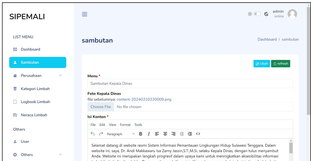
Gambar 13 Menu Sambutan
