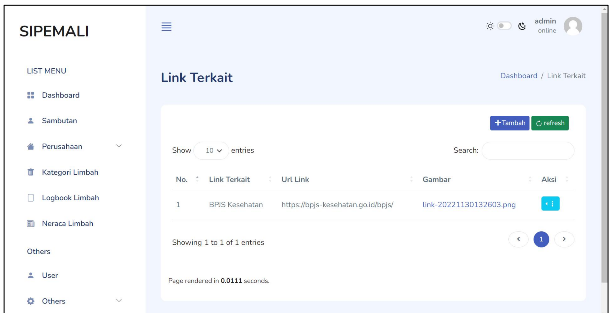
Gambar 48 Link Terkait
