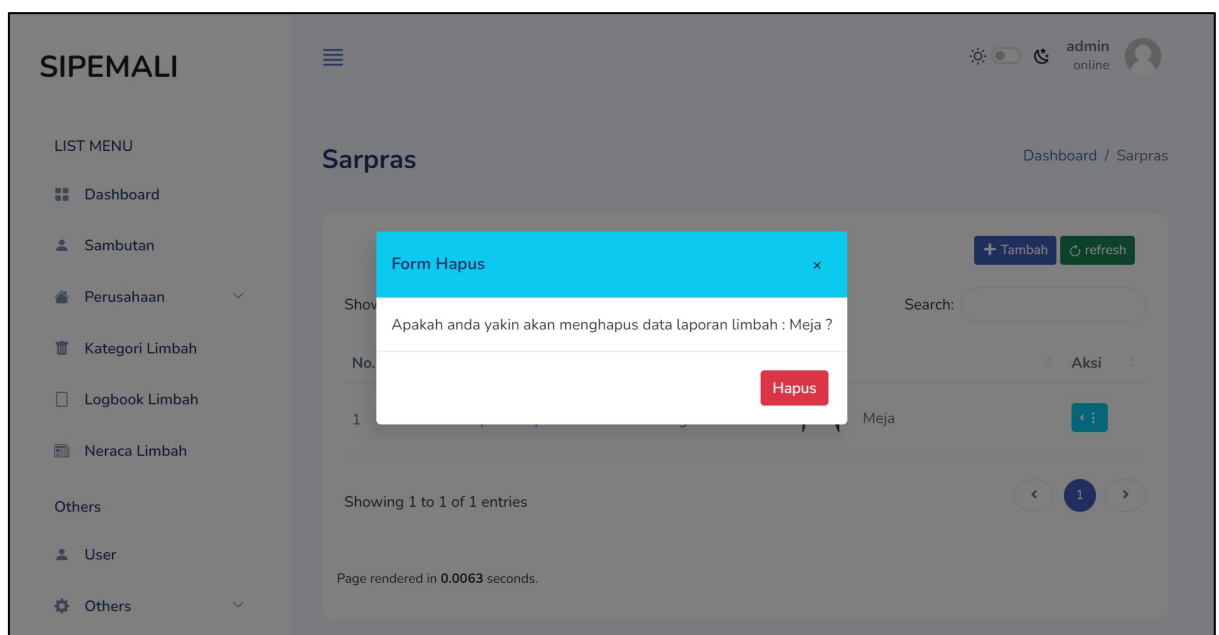
Gambar 31 Hapus Data
