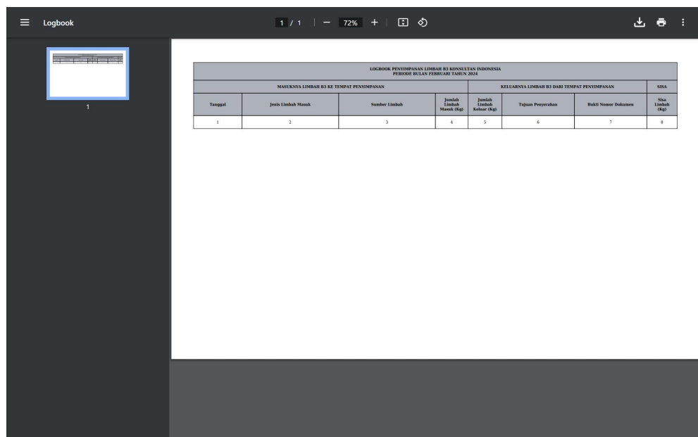
Gambar 69 Cetak Logbook
