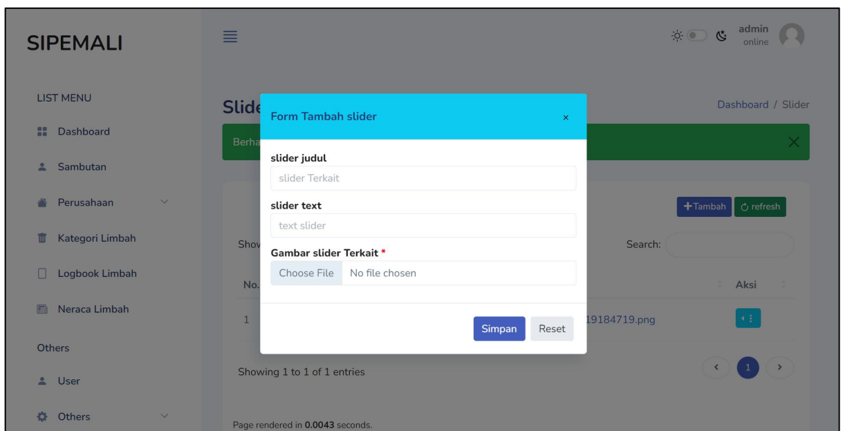
Gambar 54 Tambah data
