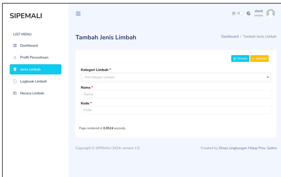
Gambar 63 Tambah data
