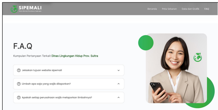
Gambar 6 FAQ
