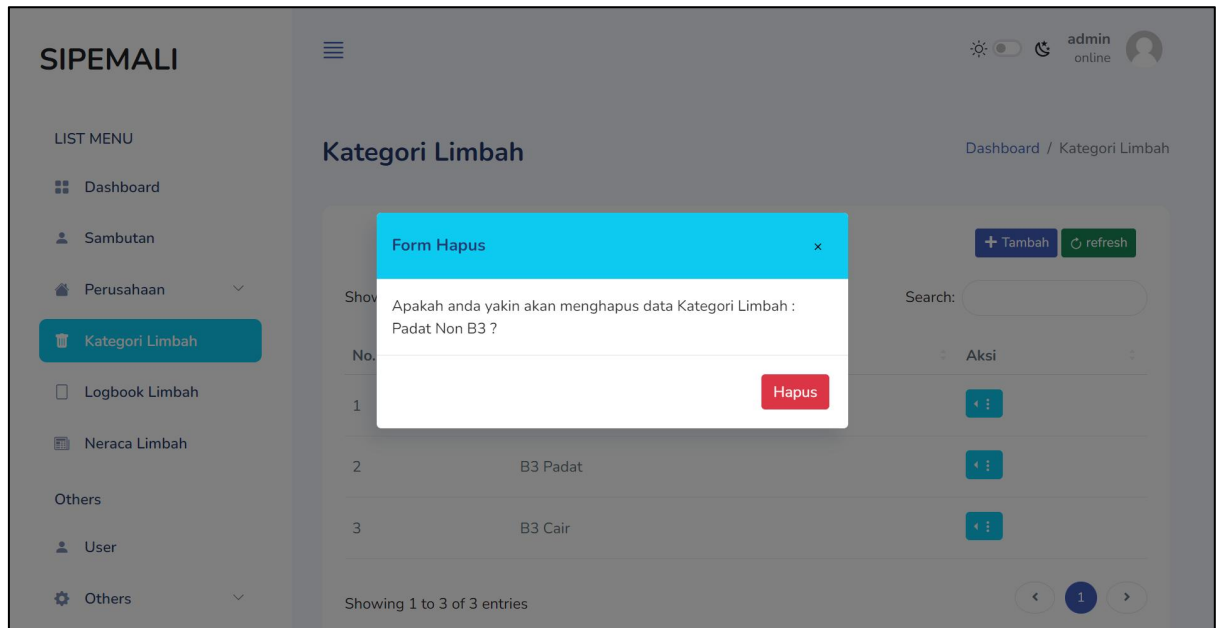
Gambar 37 Hapus Data
