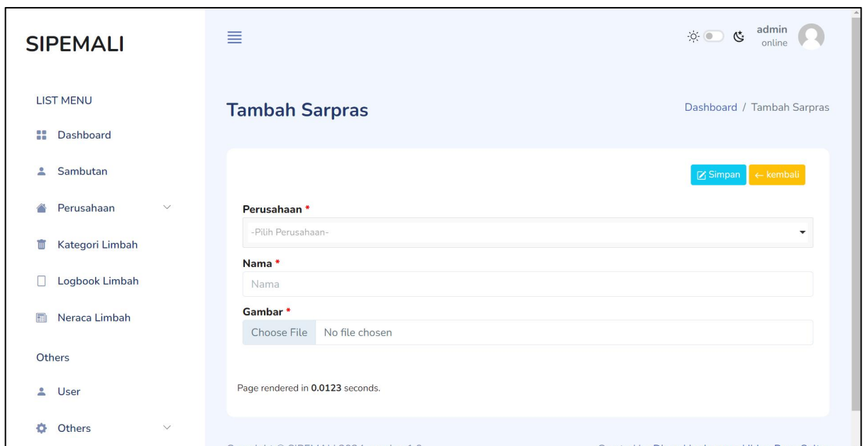
Gambar 27 Tambah Sarpra
