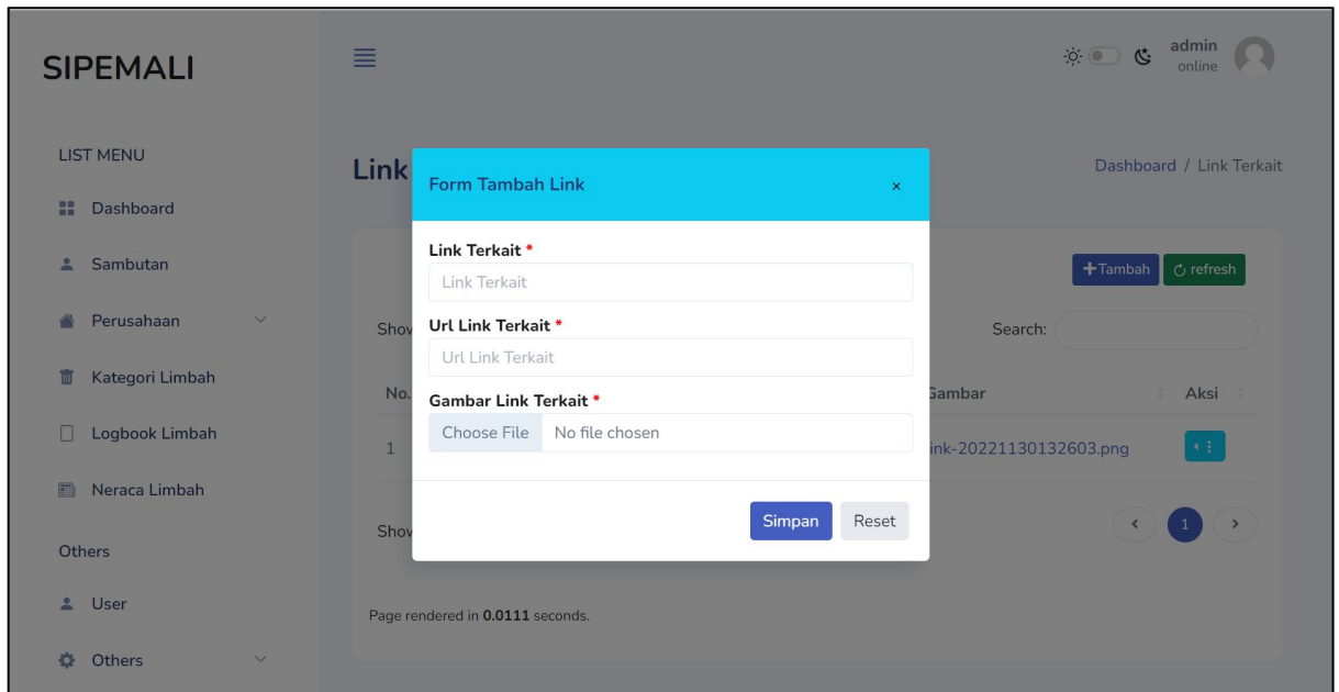
Gambar 49 Tambah data
